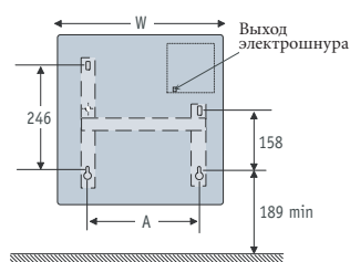
Вид спереди
